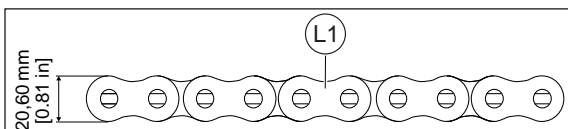
Figure 194: Usure du profil des plaques 1
