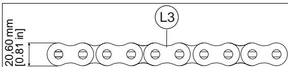
Figure 200: Usure du profil des plaques 2
