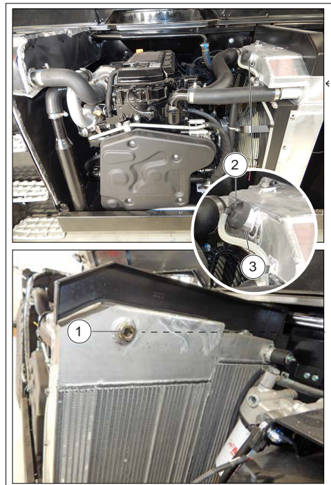
Figure 145: Niveau de liquide de refroidissement
