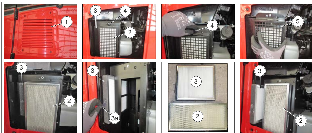
Figure 178: Vérification des filtres de ventilation de la cabine
