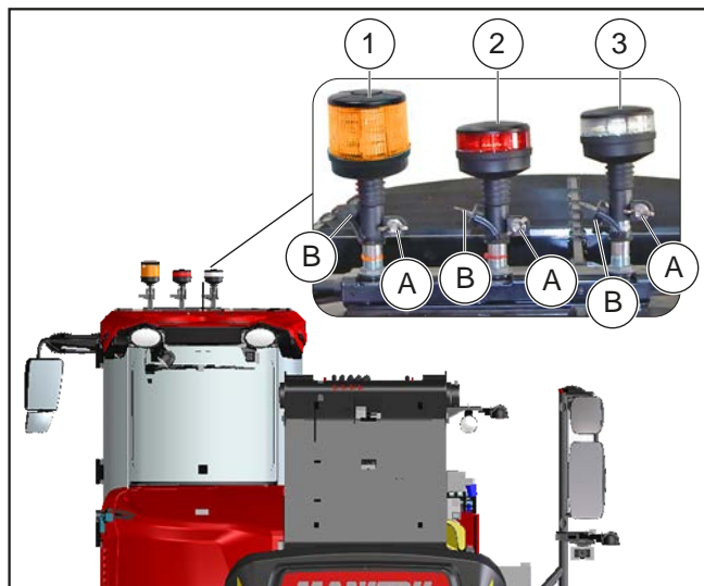
Figure 65: Phares et gyrophaire
