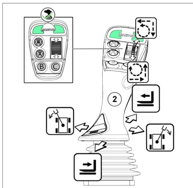
Figure 103: Manipulateur gauche
