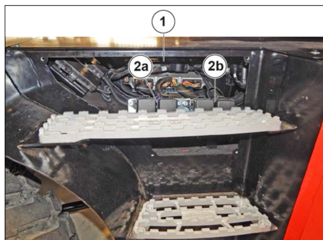
Figure 216: Fusibles et relais sur le châssis
