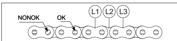
Figure 202: Alignement des épaulements des axes saillants
