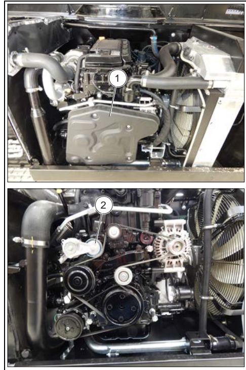
Figure 208: Remplacement de la courroie de service du moteur triphasé
