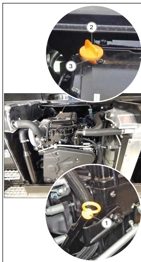
Figure 144: Niveau d'huile moteur
