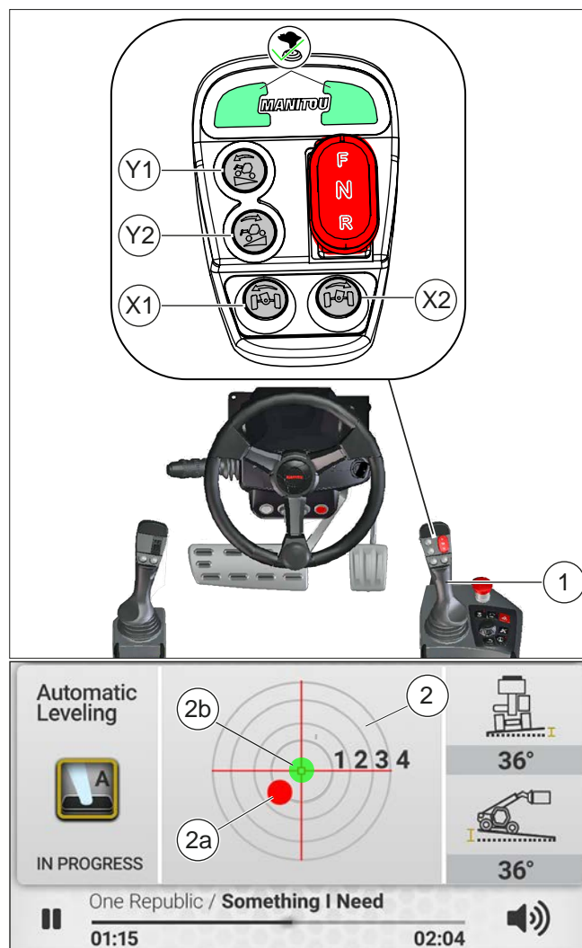
Figure 134: Procédure de nivellement (sur pneus)
