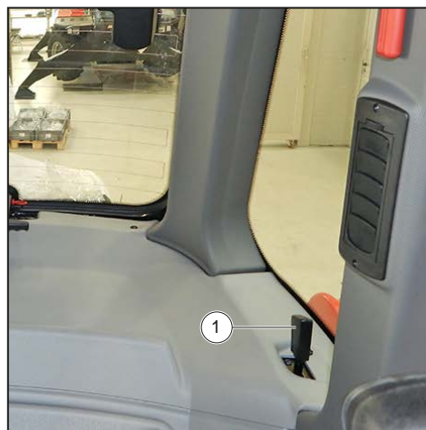
Figure 60: Levier d'ouverture de la vitre de la porte depuis l'intérieur de la cabine
