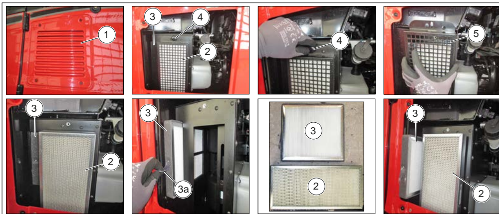
Figure 192: Remplacement des filtres de ventilation de la cabine
