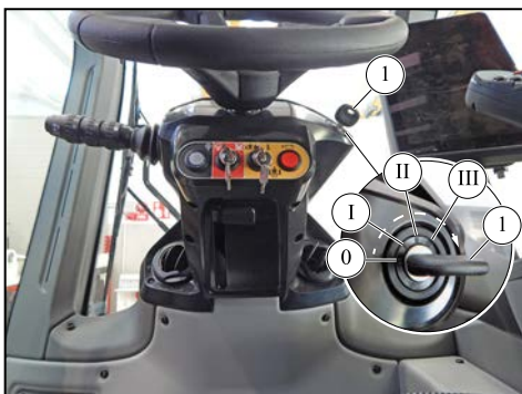
Figure 73: Contacteur à clé
