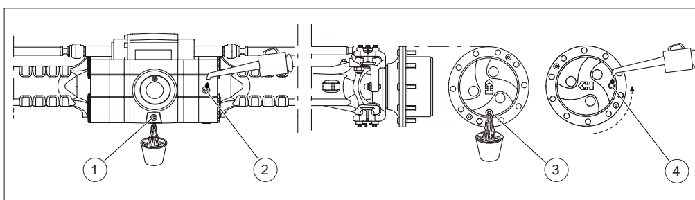
Figure 183: Changement d'huile du réducteur final des ponts avant et arrière
