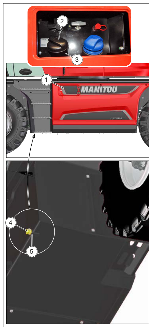
Figure 187: Nettoyage du réservoir de carburant
