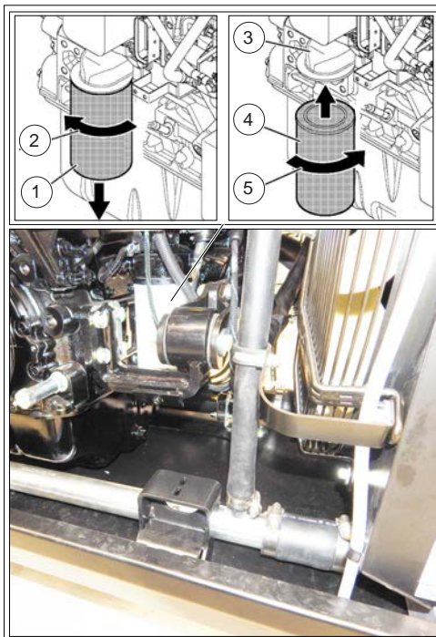
Figure 180: Remplacement du filtre à huile moteur
