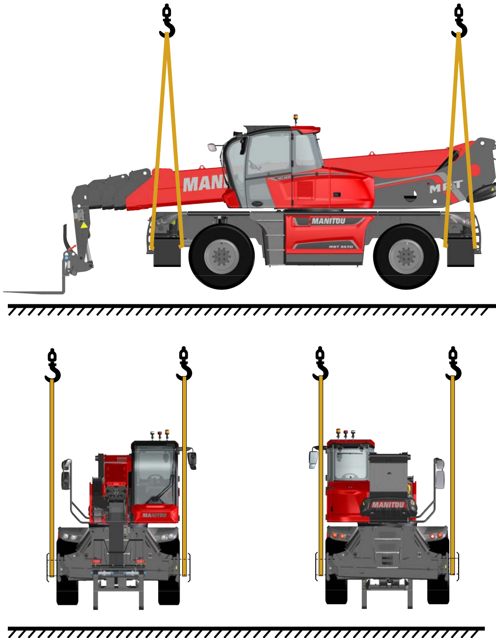
Figure 141: Mettre le chariot télescopique dans une élingue et le lever
