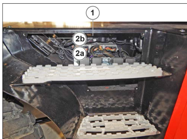
Figure 220: FUSIBLE DE LA BOÎTE D'ALIMENTATION DU CHARIOT TÉLESCOPIQUE
