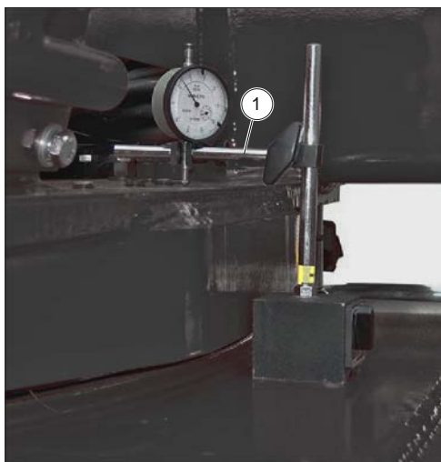
Figure 203: Vérification de l'usure et de l'augmentation du jeu des roulements de la sellette
