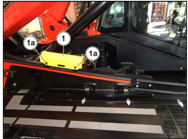
Figure 67: Cale de sécurité de la flèche
