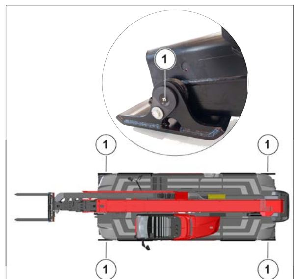
Figure 159: Nettoyage et lubrification des goupilles avant et arrière des pieds des stabilisateurs
