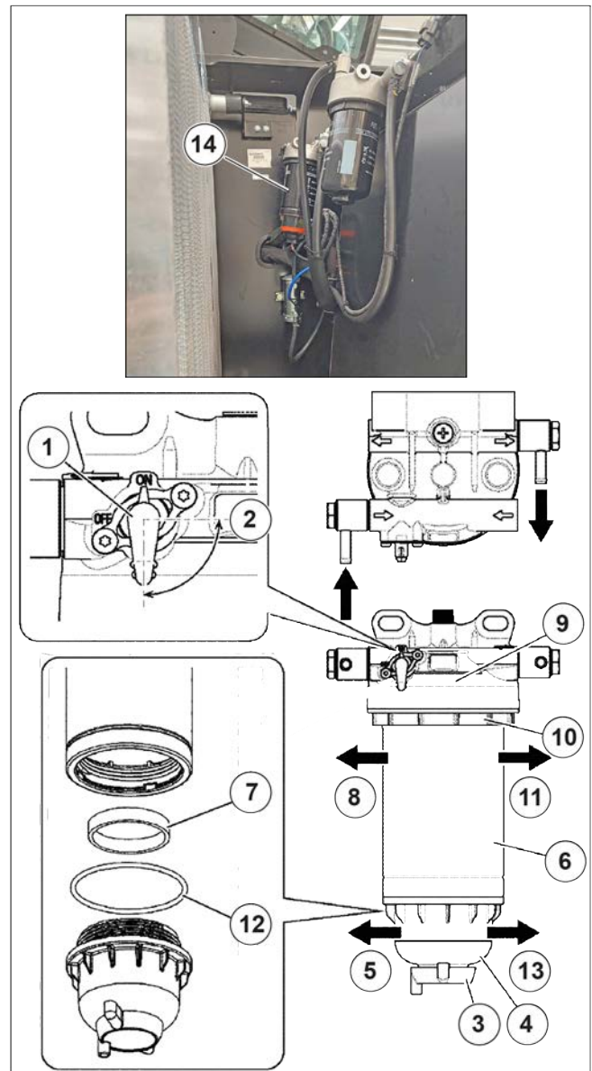
Figure 188: Remplacement du préfiltre à carburant
