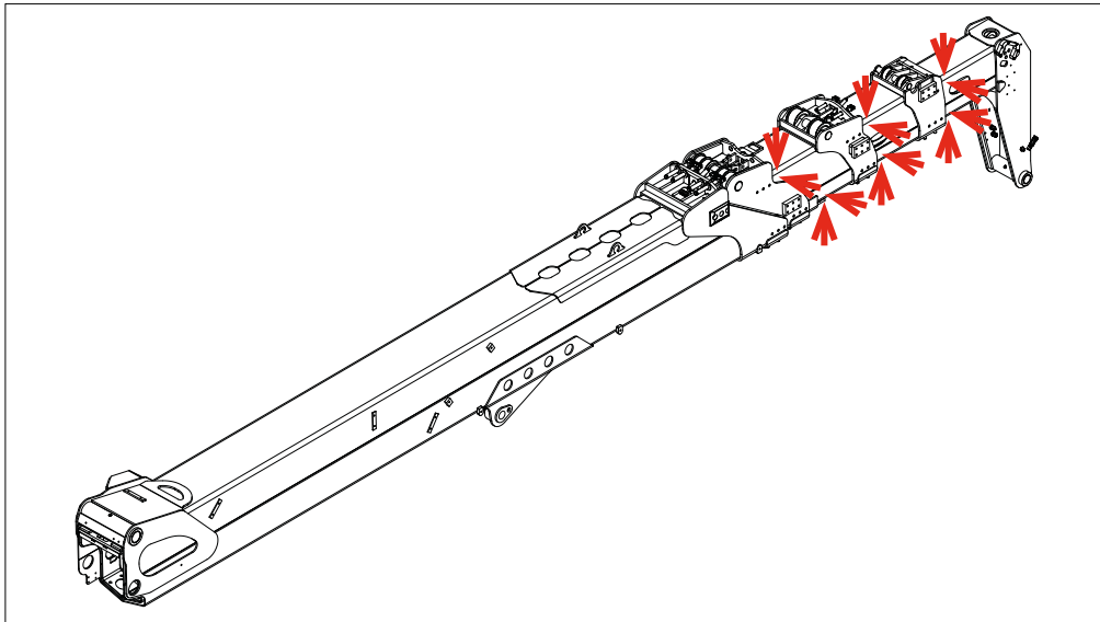
Figure 146: Patins de glissement de la flèche télescopique
