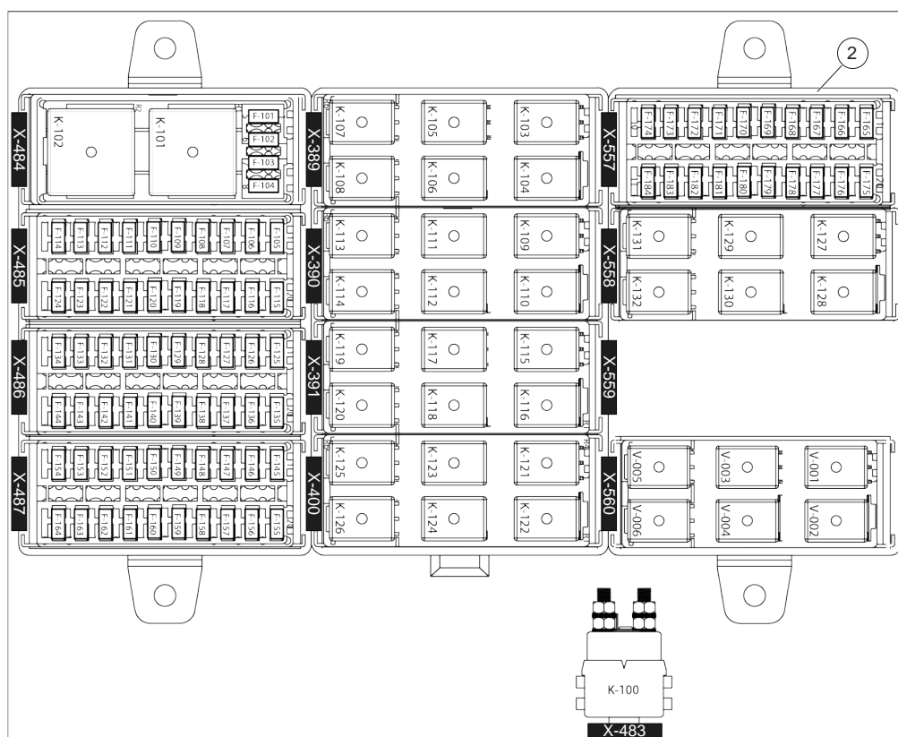
Figure 215: Aperçu des fusibles et relais
