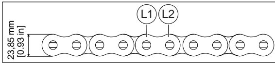
Figure 199: Usure du profil des plaques 1
