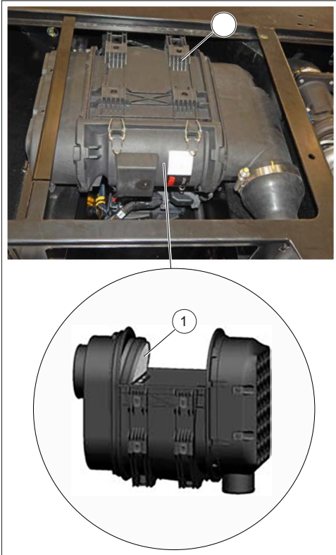
Figure 207: Remplacement de la cartouche de sécurité du filtre à air
