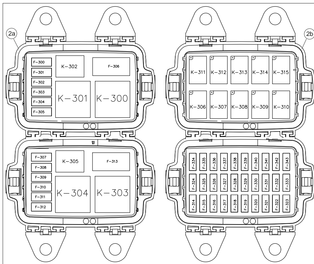
Figure 219: Aperçu des fusibles et relais :
