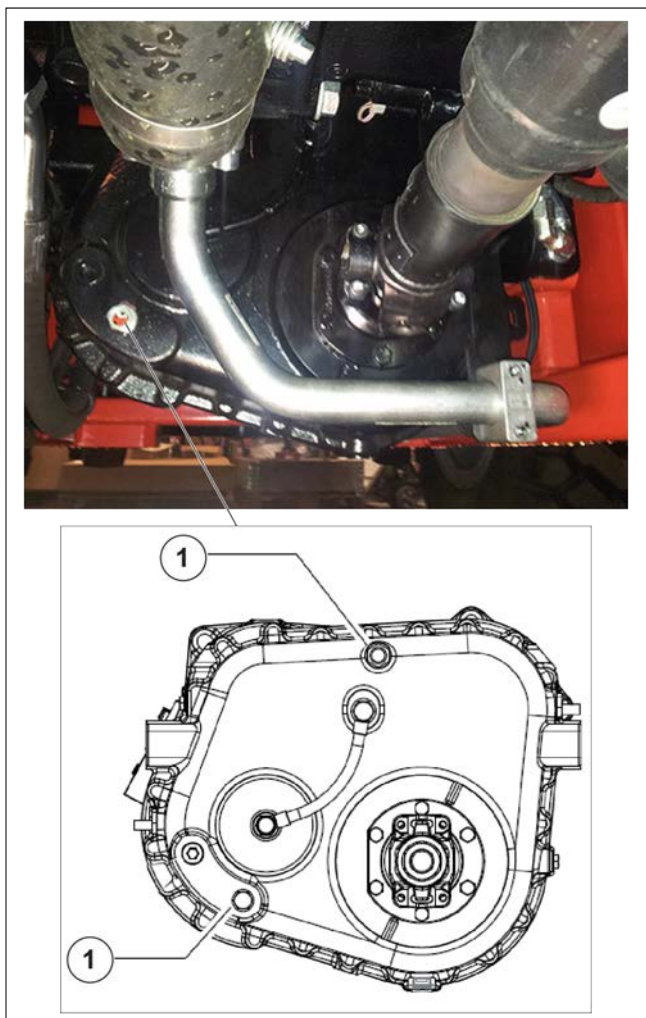
Figure 164: VÉRIFICATION DU NIVEAU D'HUILE DE LA BOÎTE DE VITESSES
