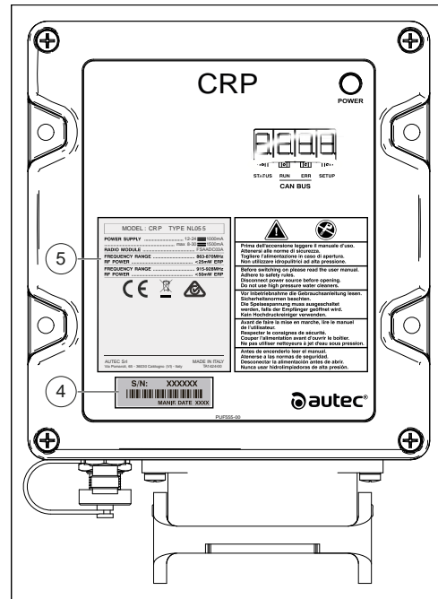
Figure 118: Plaques du récepteur
