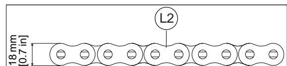
Figure 195: Usure du profil des plaques 2
