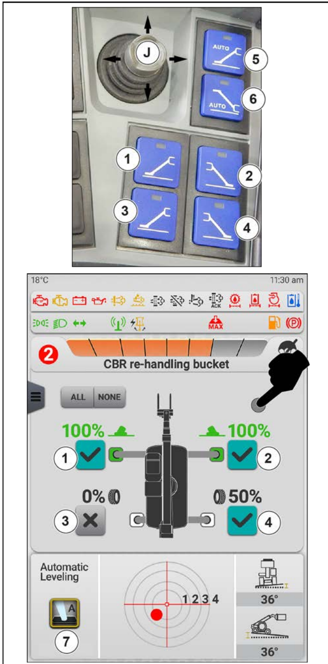
Figure 136: Procédure de nivellement automatique des stabilisateurs
