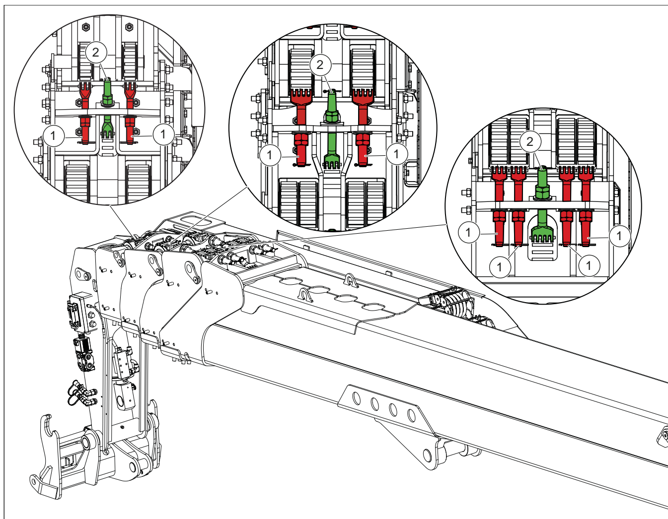
Figure 172: Réglage de la tension des chaînes T1 - T2 - T3
