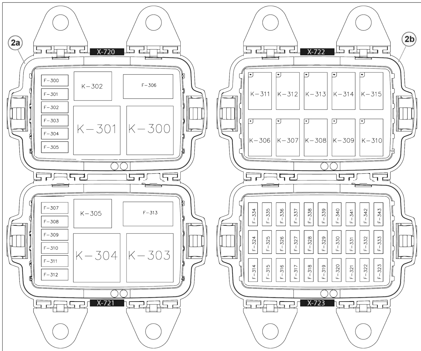
Figure 217: Aperçu des fusibles et relais :
