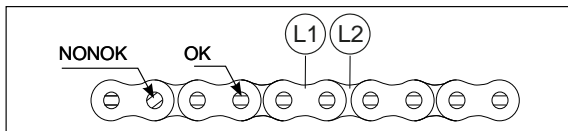
Figure 197: Alignement des épaulements des axes saillants
