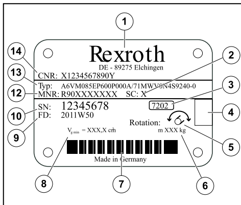
Figure 20: Plaque du moteur hydrostatique 2
