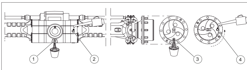
Figure 182: Changement d'huile du différentiel des ponts avant et arrière
