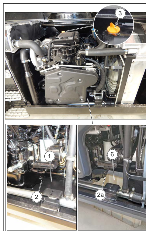
Figure 179: Vidange de l'huile moteur
