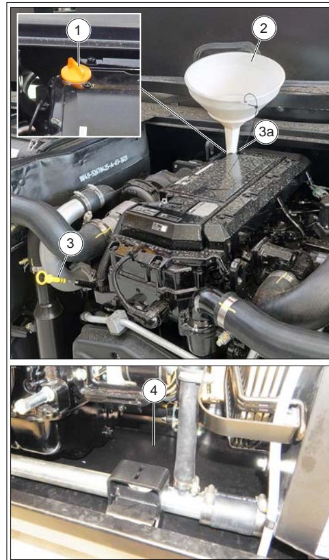
Figure 181: Remplissage d'huile moteur
