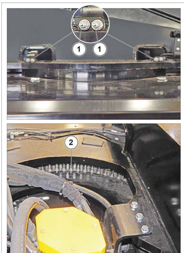
Figure 160: Nettoyage et lubrification de la sellette de rotation de la tourelle
