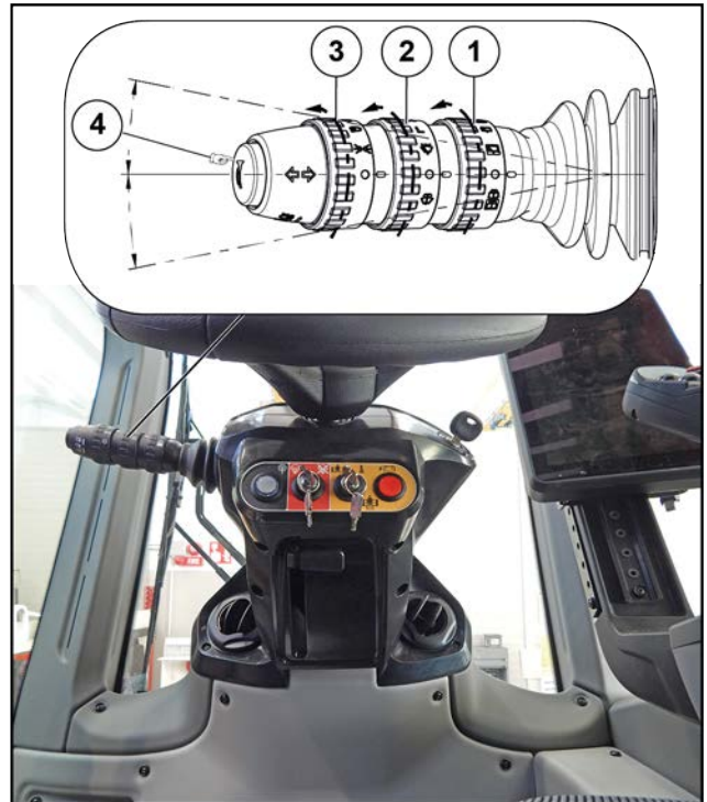
Figure 54: Levier de commande des feux, klaxon, clignotants et essuie-glaces
