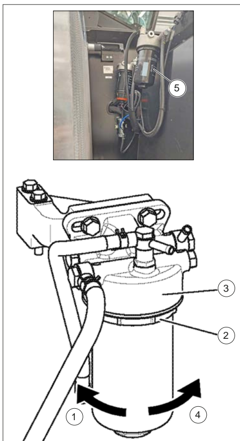
Figure 189: Remplacement du filtre à carburant
