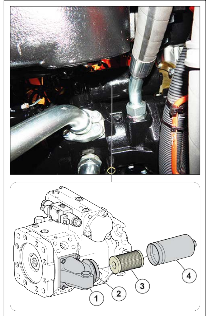
Figure 174: Remplacement du filtre à huile de la pompe hydrostatique (transmission)
