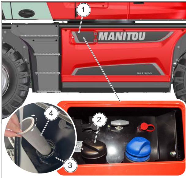
Figure 225: Vérification et nettoyage du filtre de remplissage du réservoir de carburant
