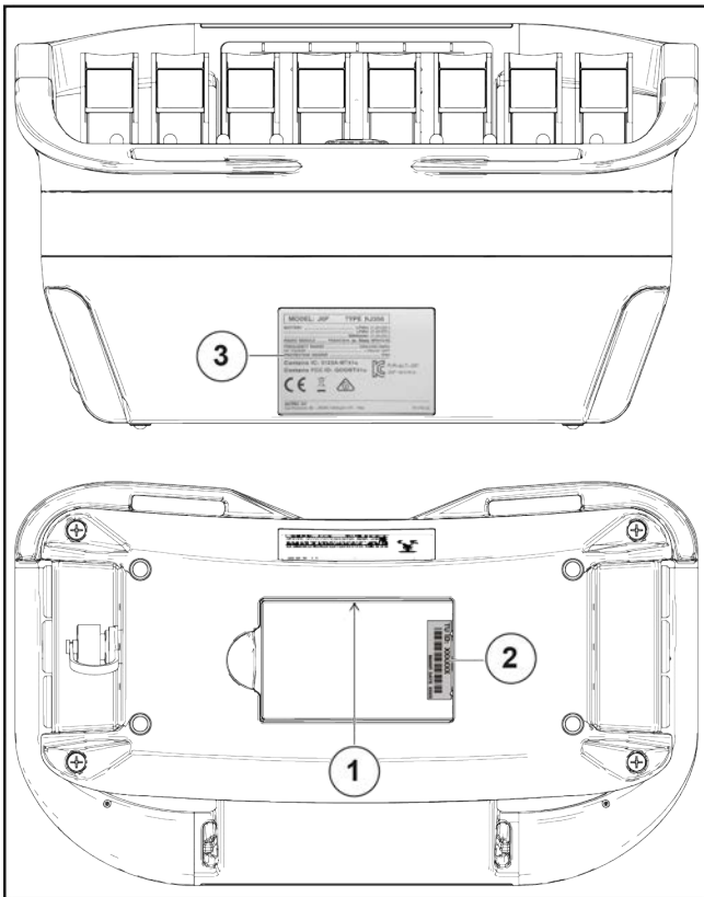
Figure 117: Plaques de l'émetteur
