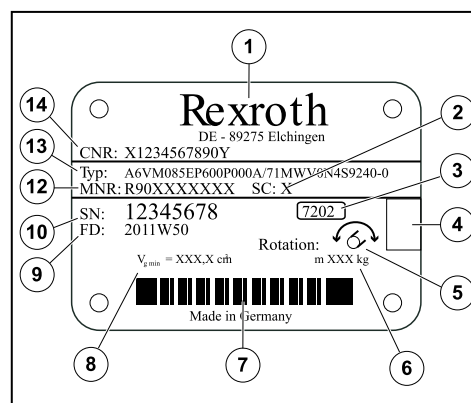
Figure 19: Plaque du moteur hydrostatique 1
