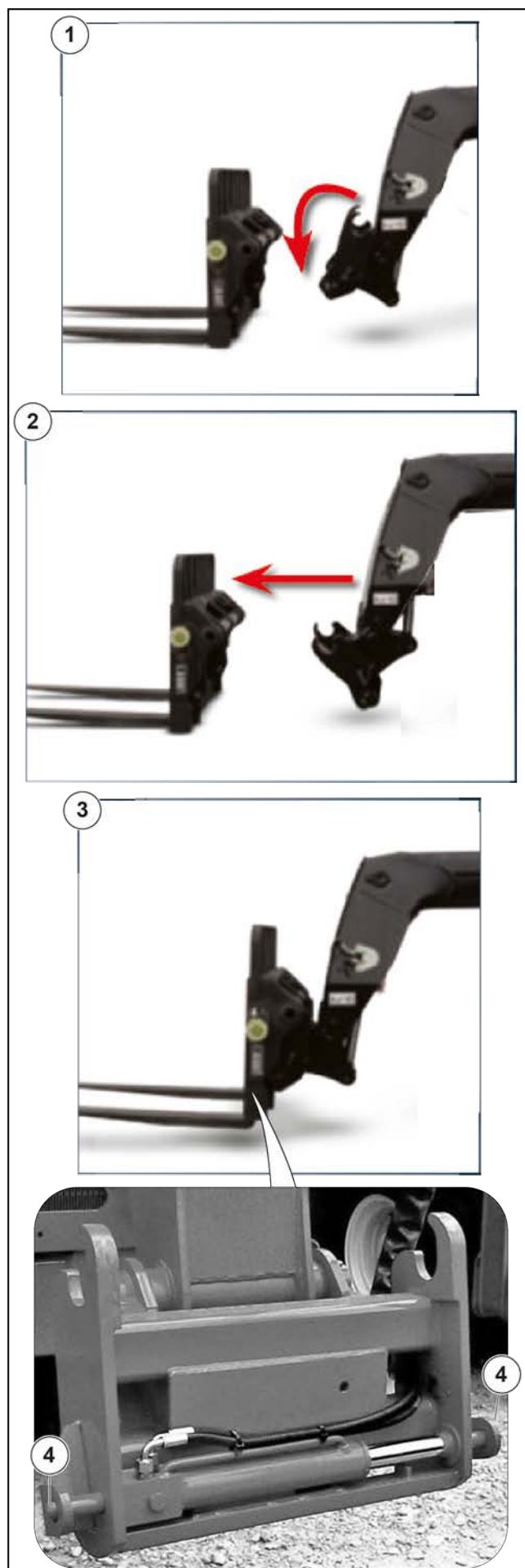
Figure 124: Repose de l'accessoire avec bloc hydraulique (en option)
