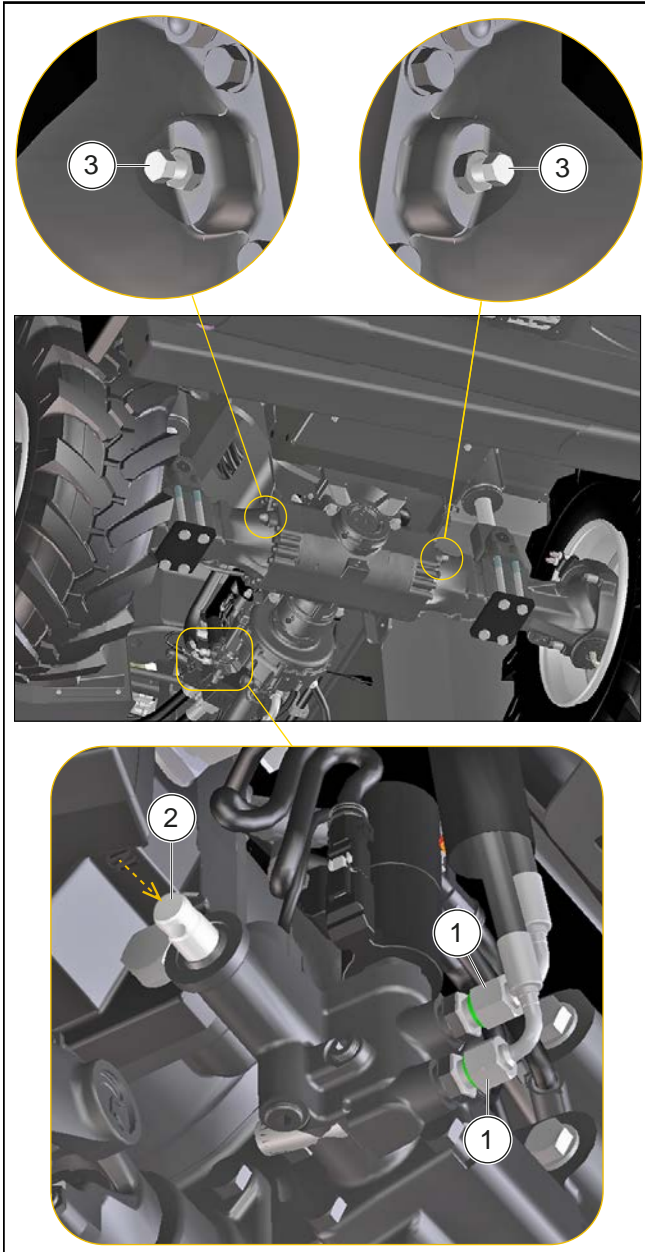
Figure 142: Remorquage ou accrochage du chariot télescopique
