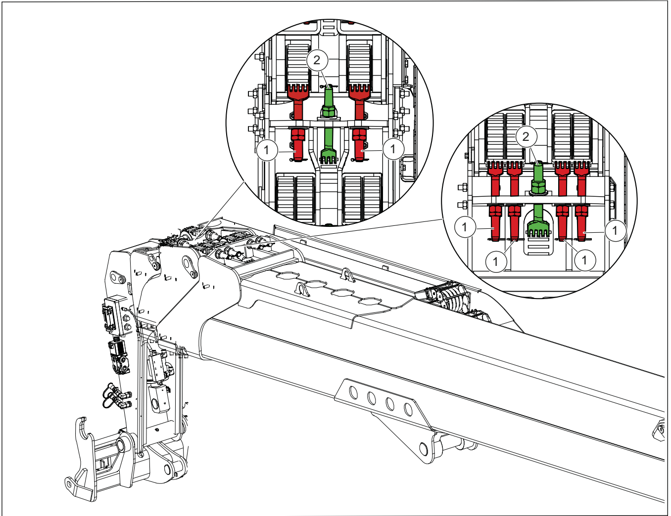
Figure 171: Réglage de la tension des chaînes T1 - T2
