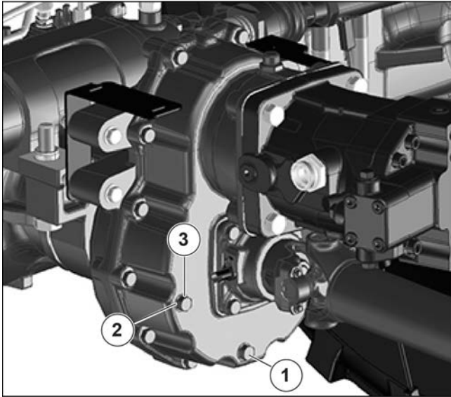
Figure 184: Changement de l'huile de la boîte de vitesses
