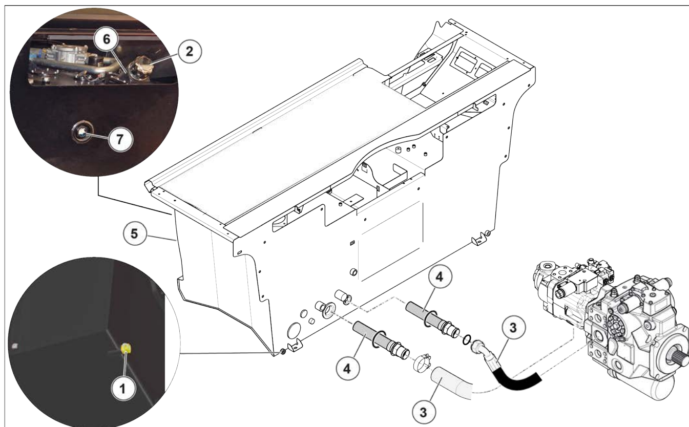
Figure 206: Remplacement de l'huile hydraulique et nettoyage de la cartouche du filtre d'admission hydraulique
