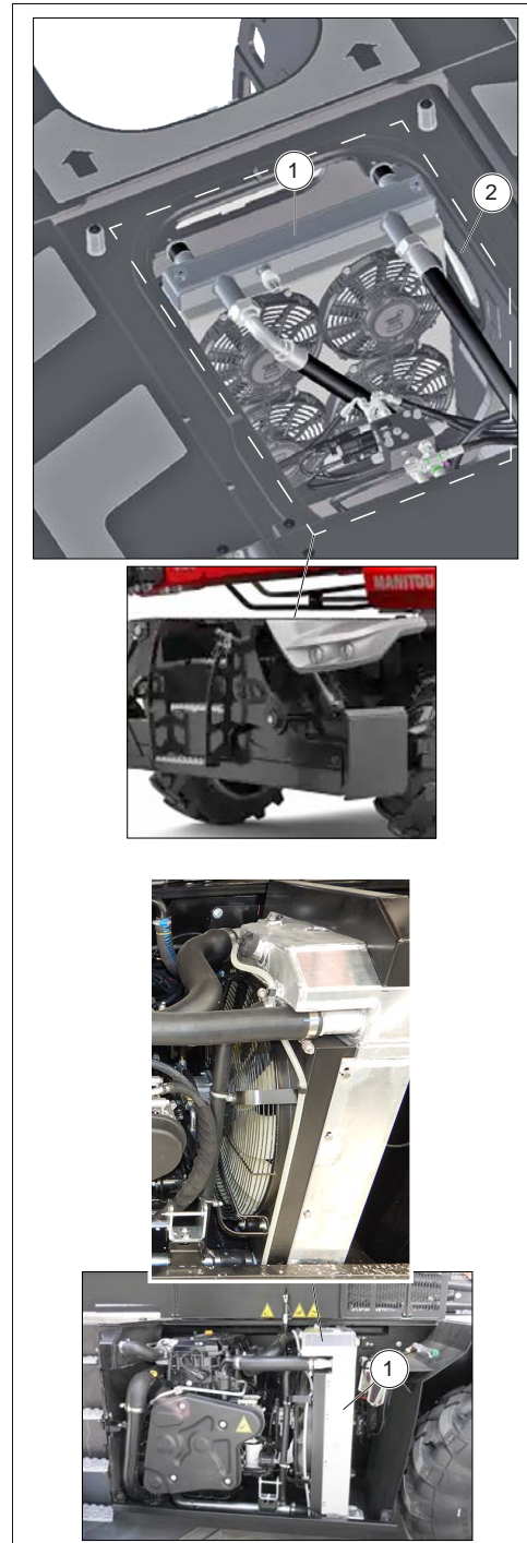
Figure 154: Nettoyage de la grille du radiateur, de l'huile hydraulique, du liquide de refroidissement et du refroidisseur
