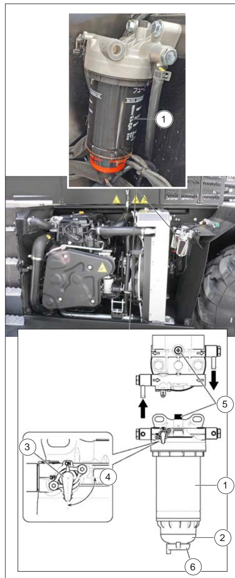
Figure 150: Vérification du préfiltre à carburant
