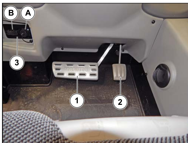
Figure 52: Pédales et prises de diagnostic
