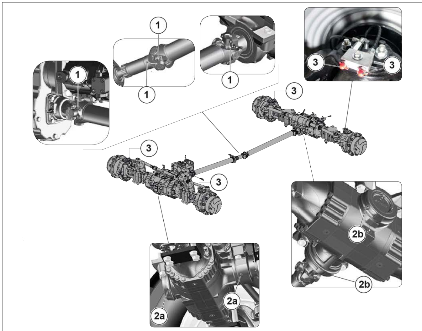
Figure 157: Lubrification des joints de cardan, de l'oscillation du pont et des goupilles des réducteurs
