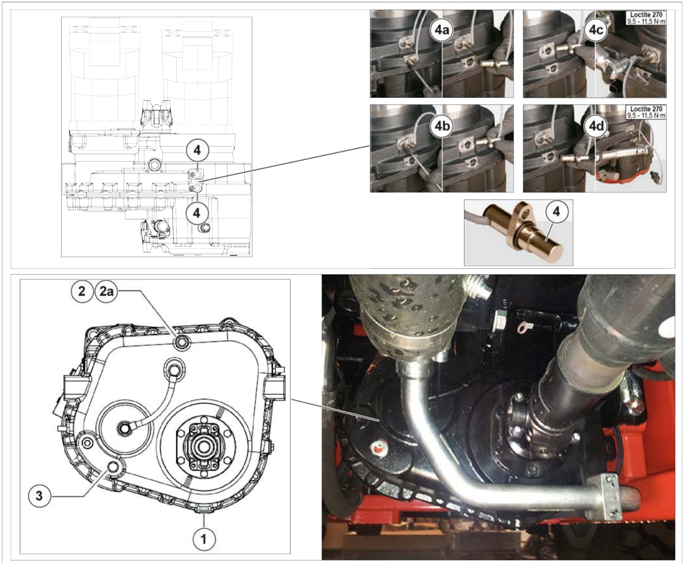
Figure 185: Changement de l'huile de la boîte de vitesses et nettoyage du capteur de vitesse
