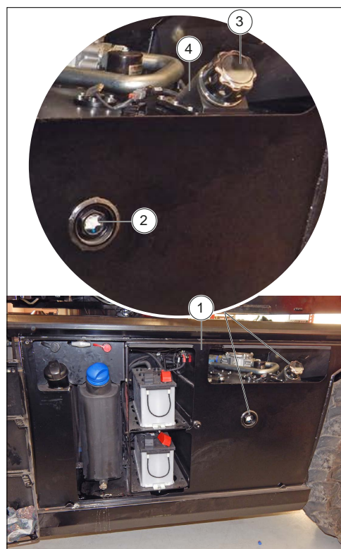
Figure 153: Vérification du niveau d'huile hydraulique
