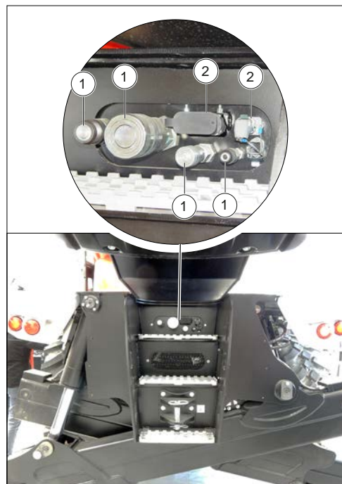
Figure 120: Préparation de l'unité bi-énergie
