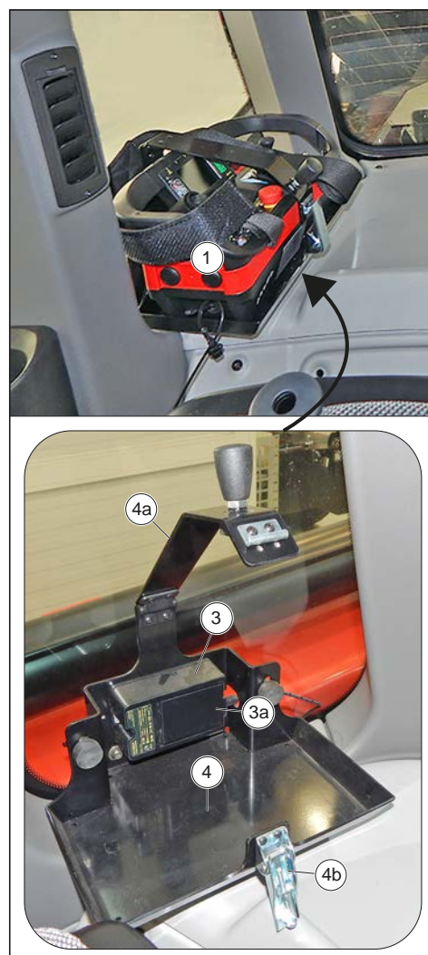
Figure 116: Émetteur et support
