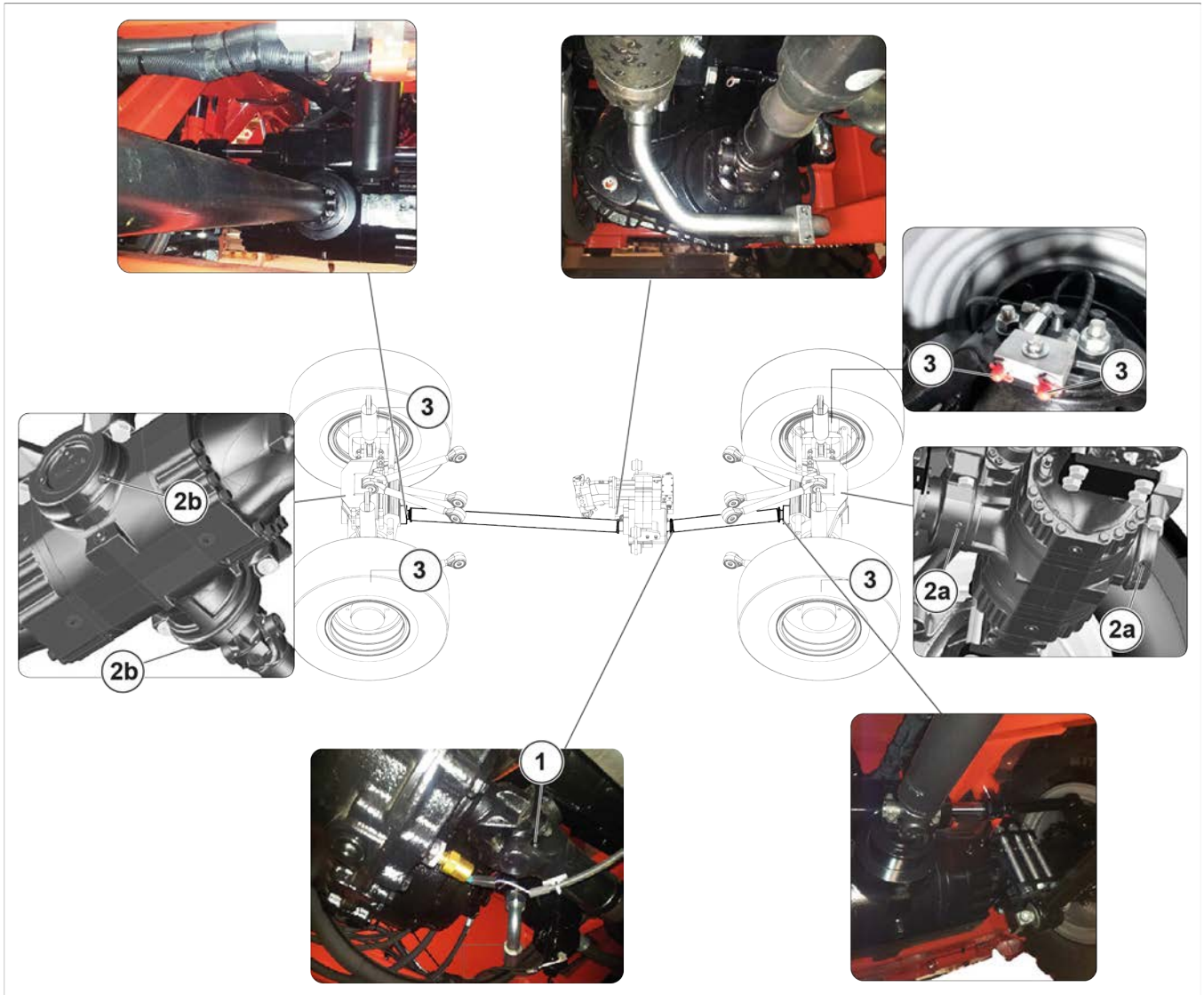
Figure 158: Lubrification des joints de cardan, de l'oscillation du pont et des goupilles des réducteurs
