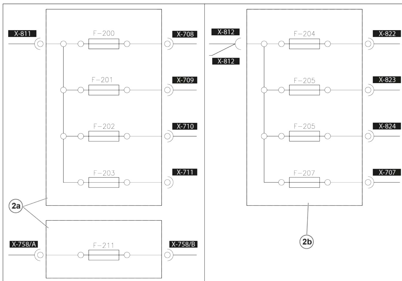
Figure 221: Aperçu des fusibles et relais :
