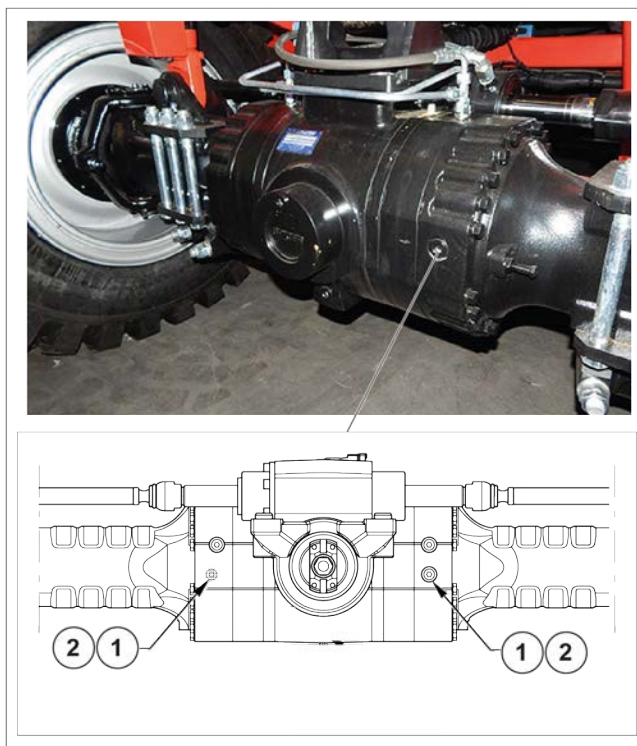
Figure 161: Vérification du niveau d'huile du différentiel des ponts avant et arrière
