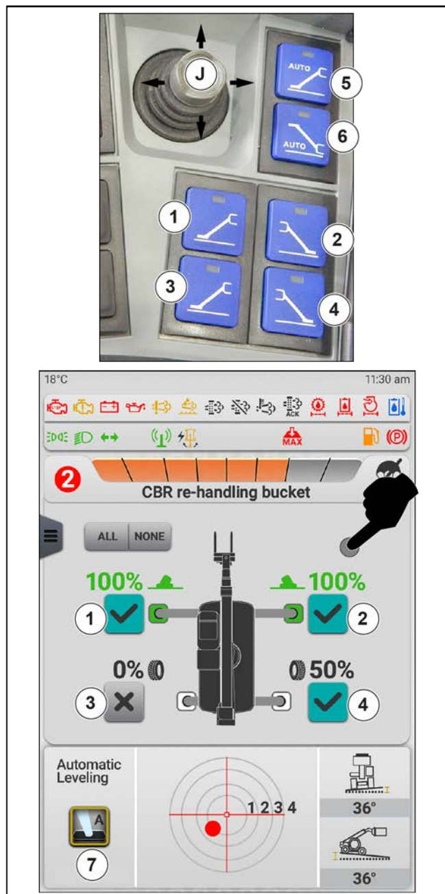
Figure 135: Procédure de stabilisation manuelle
