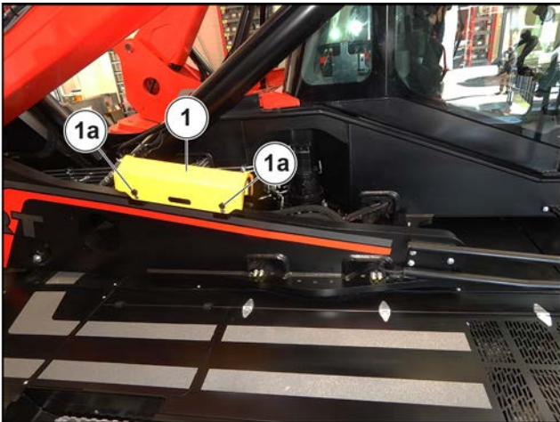
Figure 210: Cale de sécurité de la flèche
