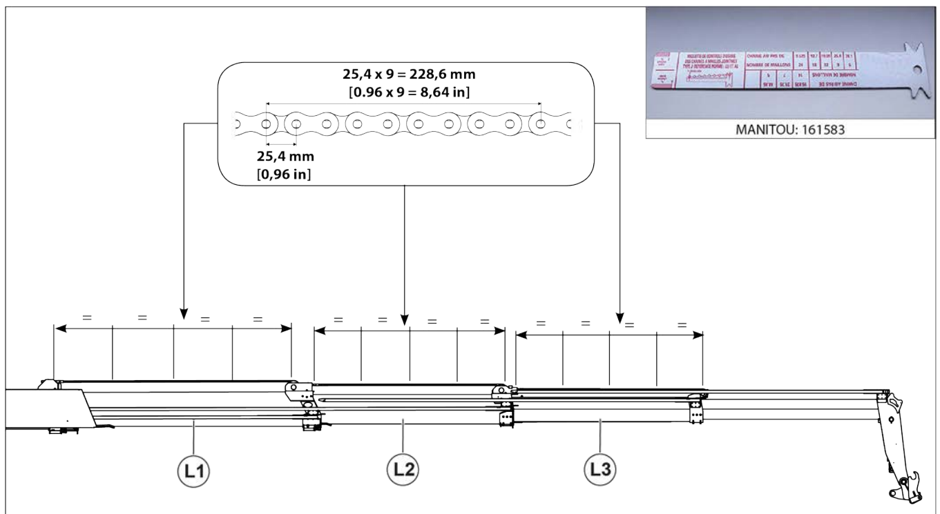
Figure 198: Allongement des chaînes
