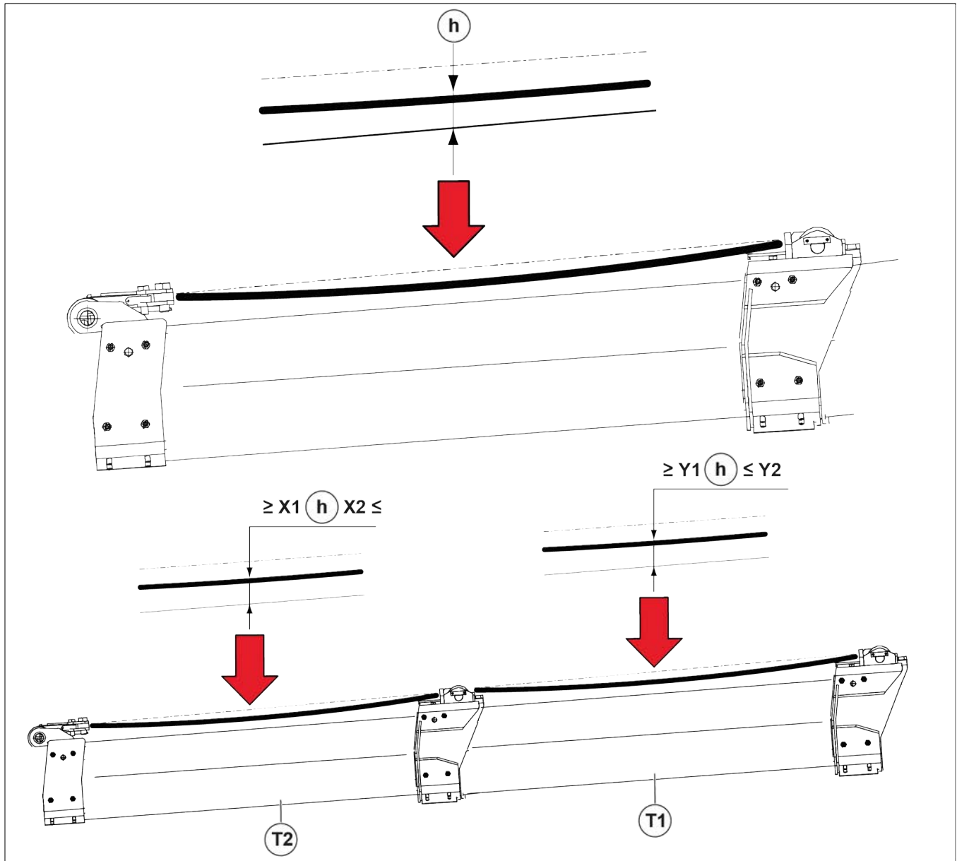
Figure 169: Contrôle de la tension des chaînes T1 - T2
