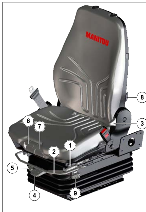
Figure 70: Siège pneumatique pour le conducteur (en option)
