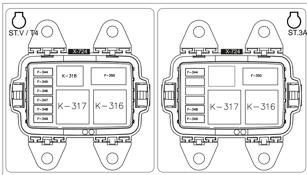
Figure 223: Aperçu des fusibles et relais :
