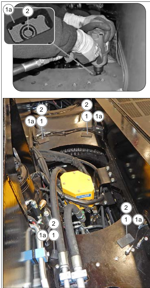
Figure 177: Vérification des boulons de fixation de la sellette et de la tourelle
