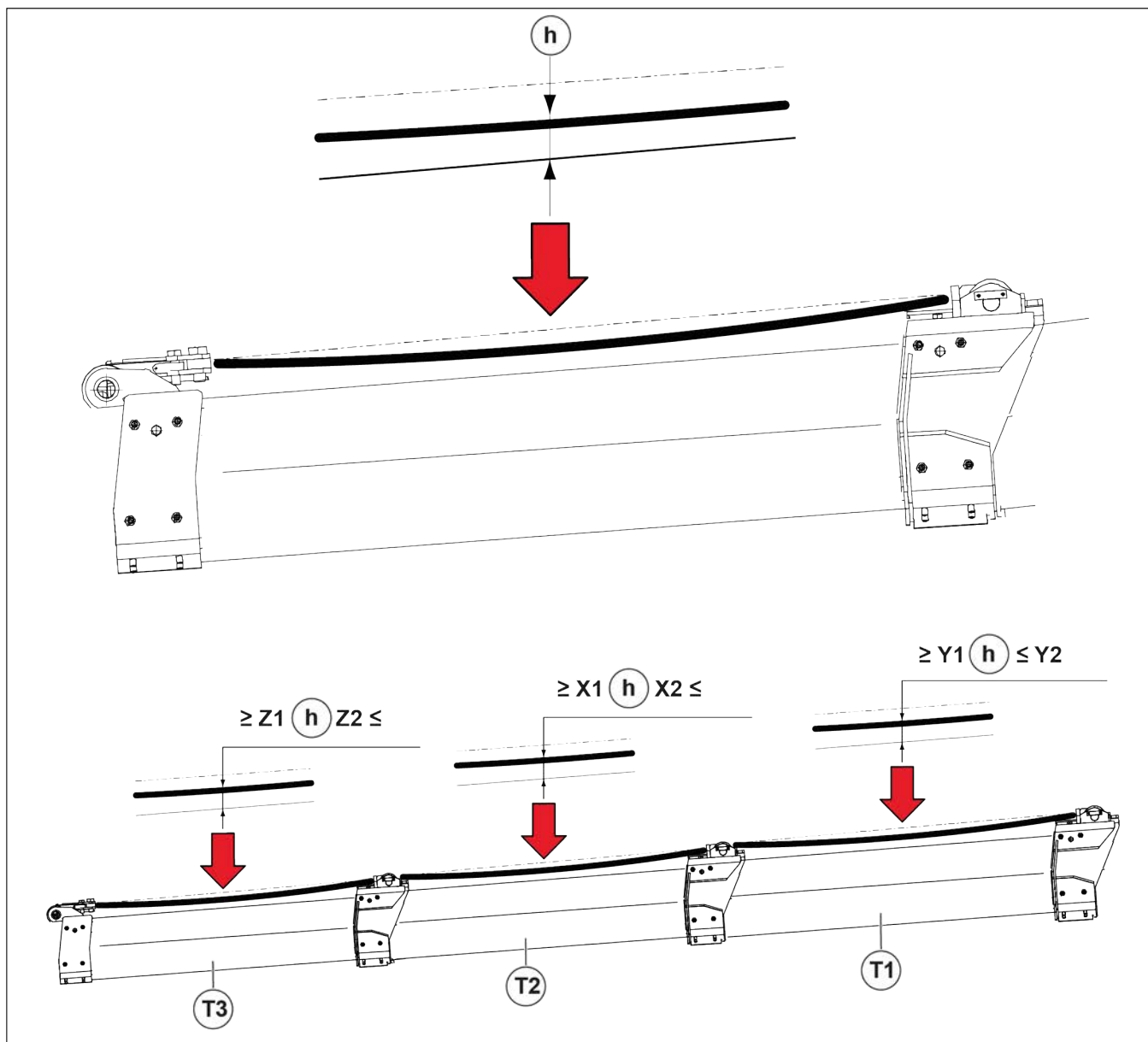
Figure 170: Contrôle de la tension des chaînes T1 - T2 - T3
