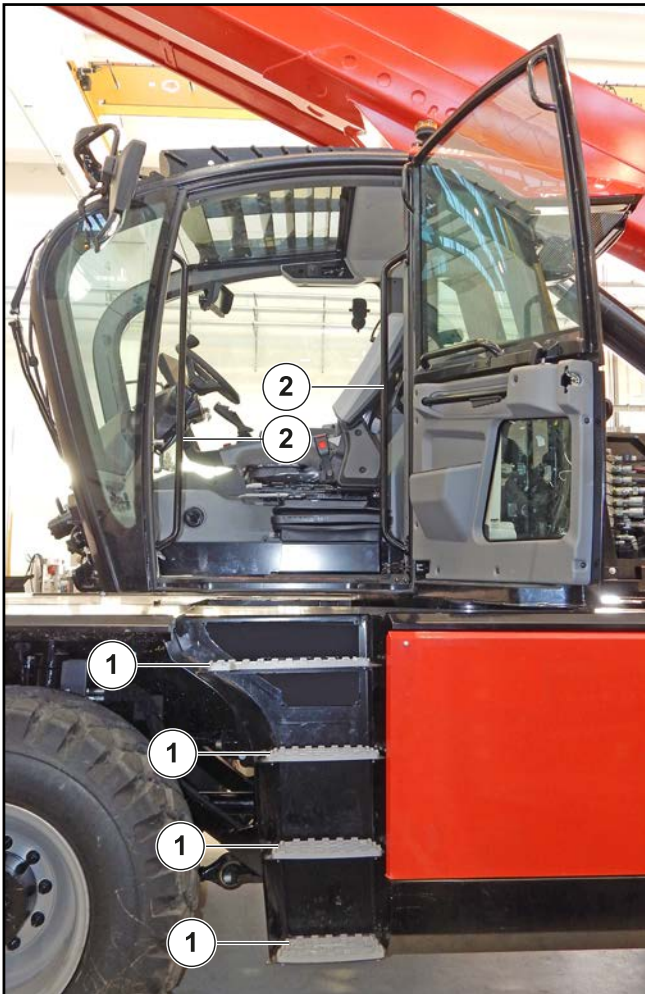
Figure 123: Montée et sortie du véhicule
