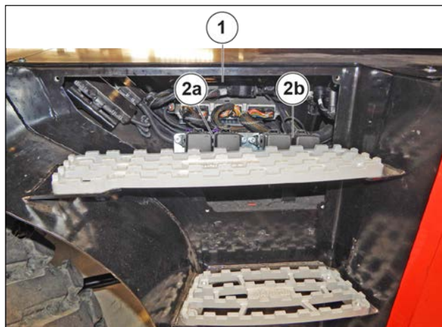
Figure 218: Fusibles et relais sur le châssis
