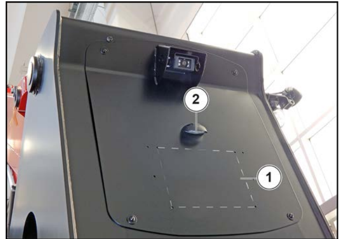
Figure 63: Plaque d'immatriculation et éclairage de la plaque
