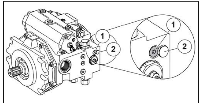
Figure 143: Dérivation de la pompe hydrostatique
