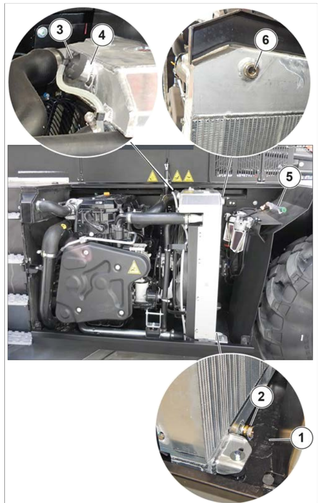
Figure 191: Remplacement du liquide de refroidissement
