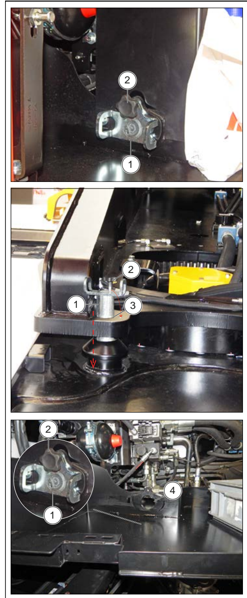
Figure 139: Blocage de la rotation de la tourelle
