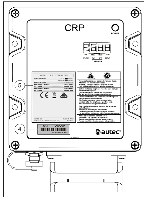
Figure 109: Plaques du récepteur
