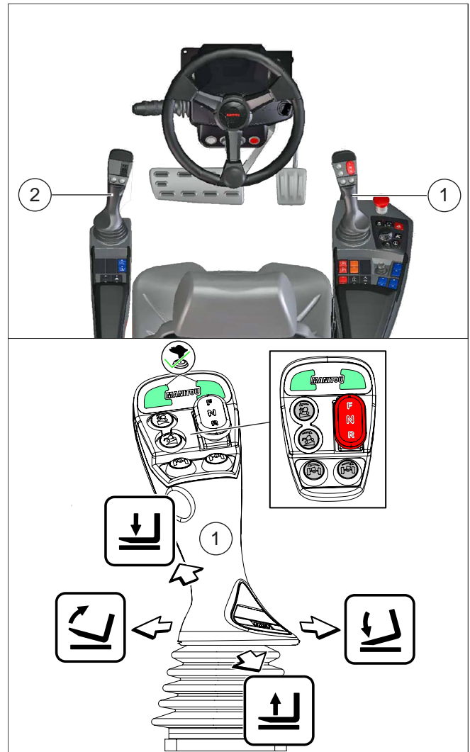
Figure 102: Manipulateur droit
