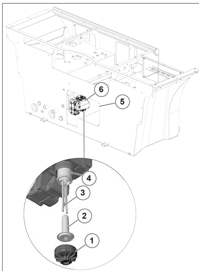
Figure 204: Remplacement du filtre de la pompe de gavage « DEF »
