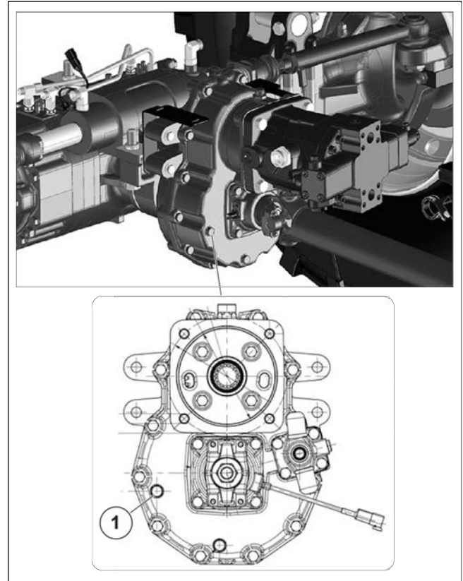
Figure 163: VÉRIFICATION DU NIVEAU D'HUILE DE LA BOÎTE DE VITESSES
