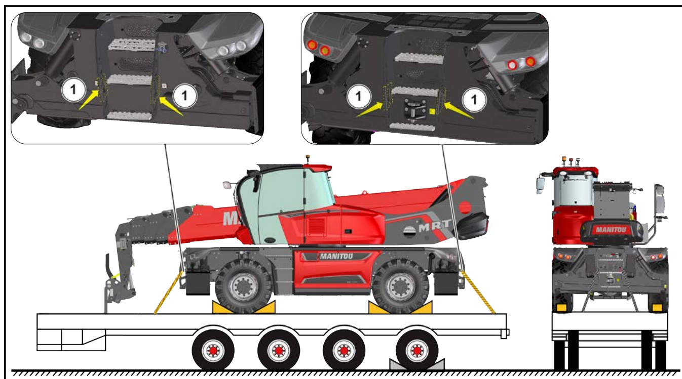
Figure 140: Mettre le chariot télescopique dans une élingue
