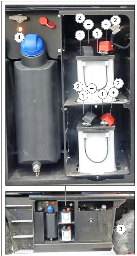
Figure 165: Vérification de la batterie
