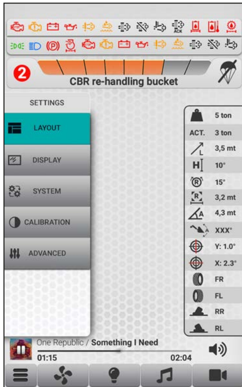
Figure 95: Page « RÉGLAGES »
