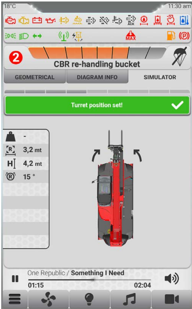
Figure 88: Onglet « SIMULATEUR »
