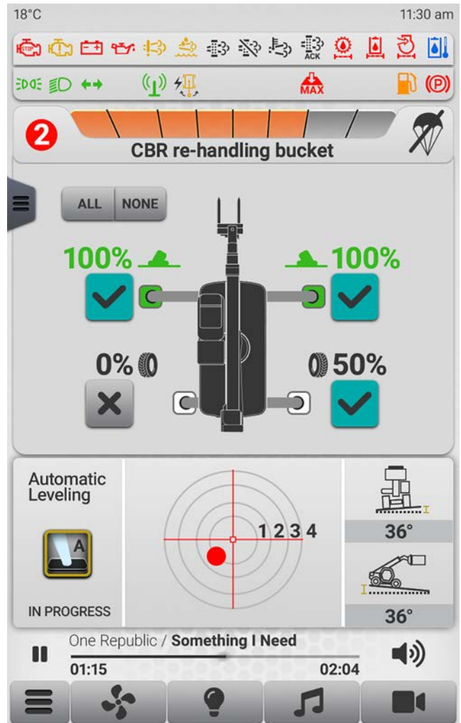
Figure 89: Page « STABILITÉ »
