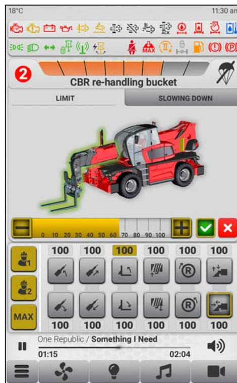
Figure 91: Onglet « RALENTISSEMENT »
