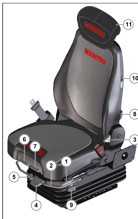
Figure 71: Siège chauffé/climatisé du conducteur (en option)
