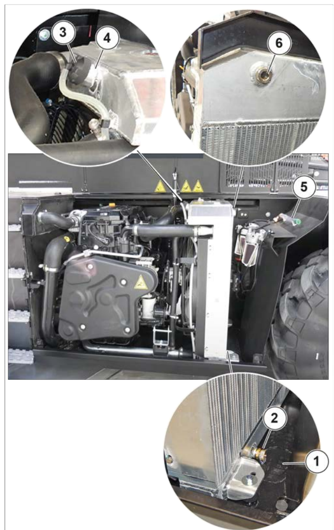
Figure 191: Remplacement du liquide de refroidissement
