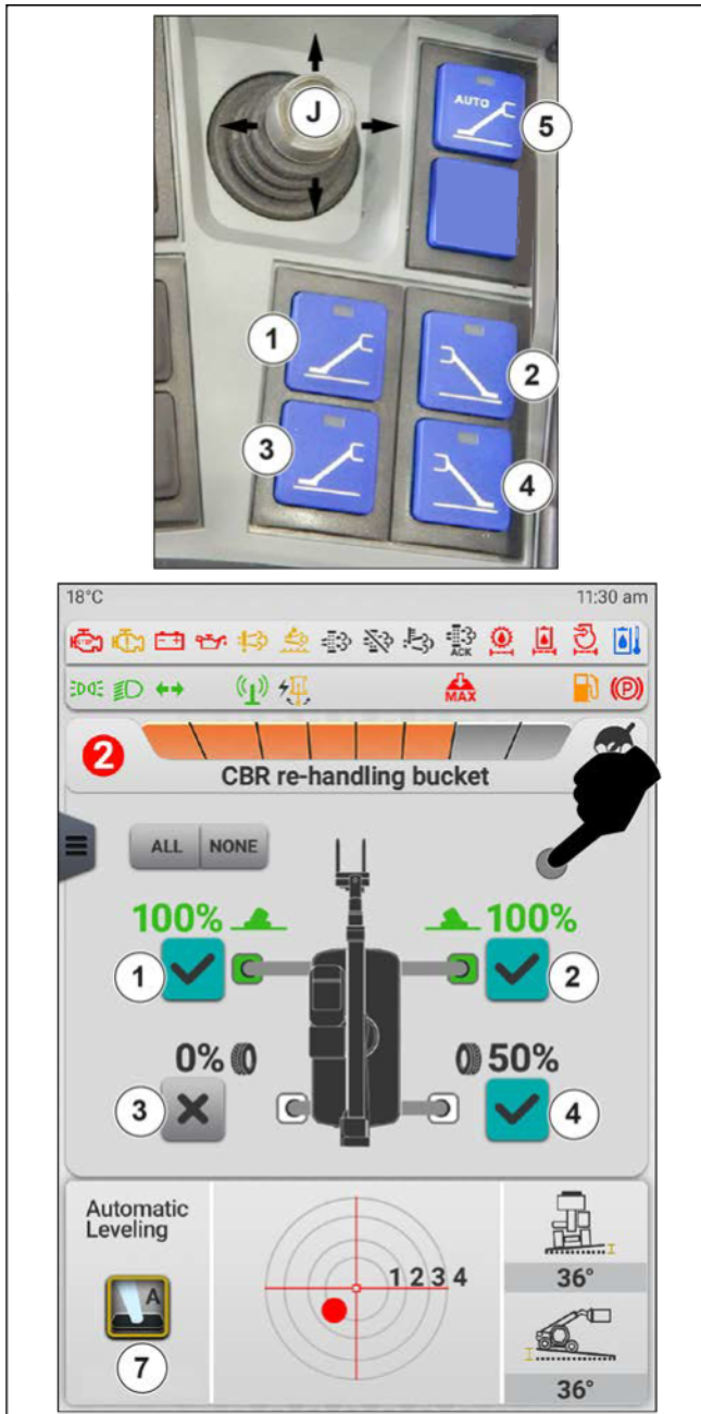
Figure 135: Procédure de stabilisation manuelle
