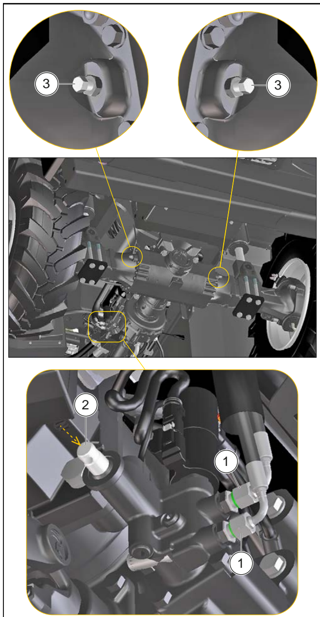
Figure 142: Remorquage ou accrochage du chariot télescopique
