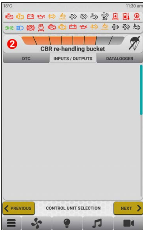
Figure 93: Onglet ENTRÉE/SORTIES
