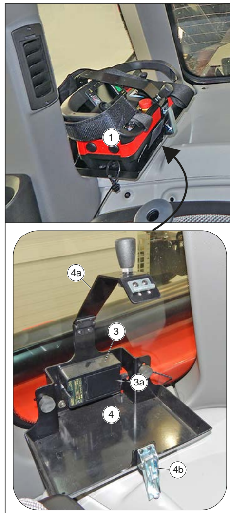
Figure 107: Unité d'émission et support
