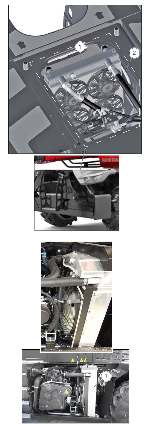
Figure 154: Nettoyage de la grille du radiateur, de l'huile hydraulique, du liquide de refroidissement et du refroidisseur
