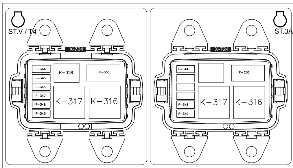
Figure 223: Aperçu des fusibles et relais :
