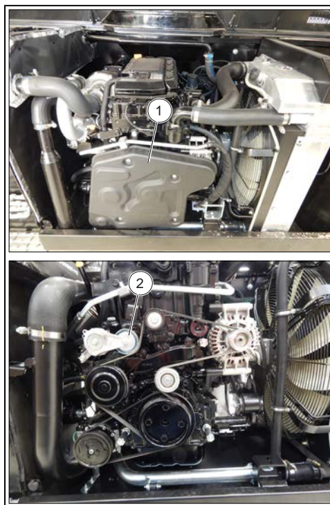
Figure 208: Remplacement de la courroie de service du moteur triphasé
