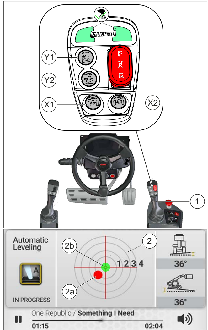
Figure 134: Procédure de nivellement (sur pneus)
