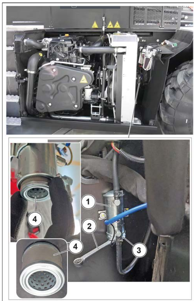
Figure 190: Remplacement du filtre de la pompe à carburant
