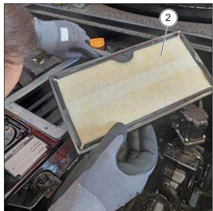
Figure 209: Remplacement du filtre du carter du reniflard du moteur
