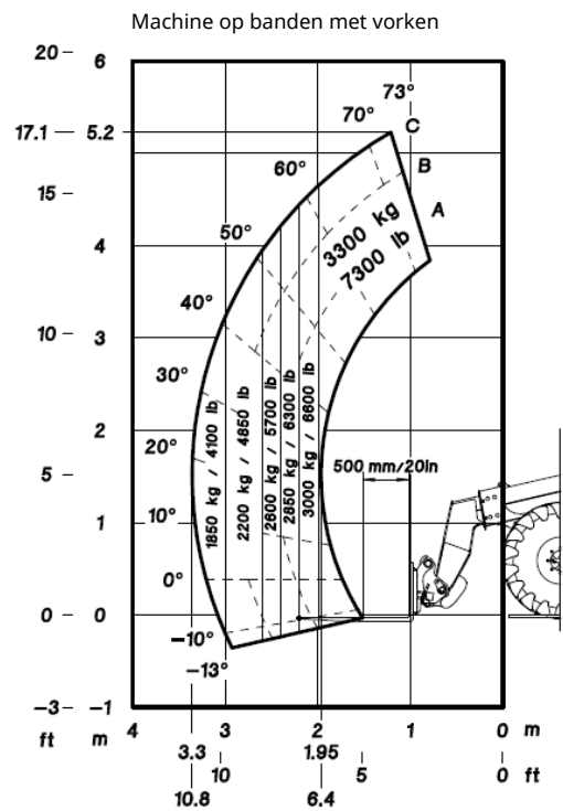
Draagvermogenstabel in overeenstemming met EN 474-3
