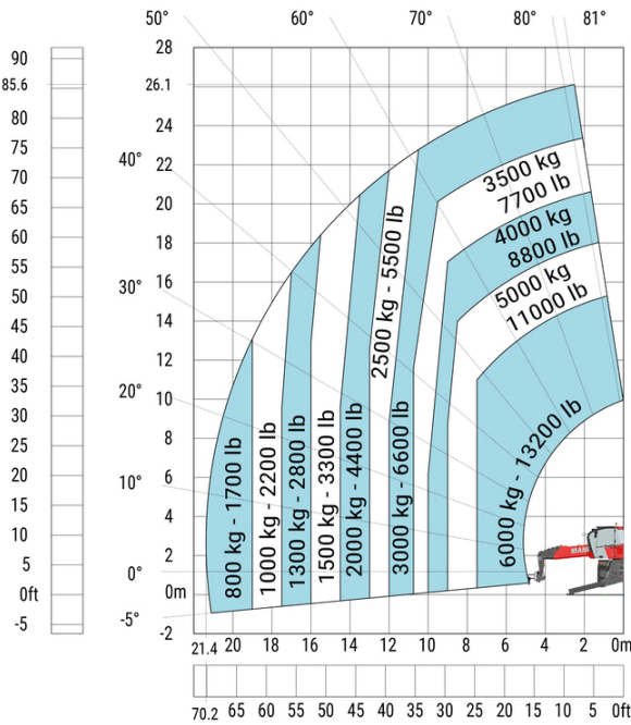
Machine op verlaagde stabilisatoren met haak 6000 kg (metrisch)
